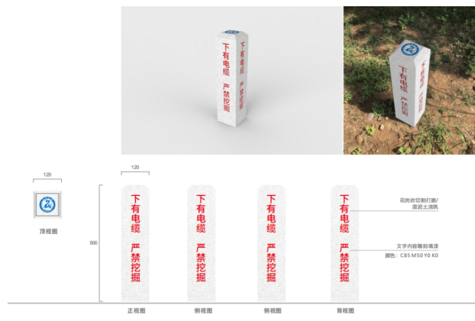
电缆桩制作标准图
