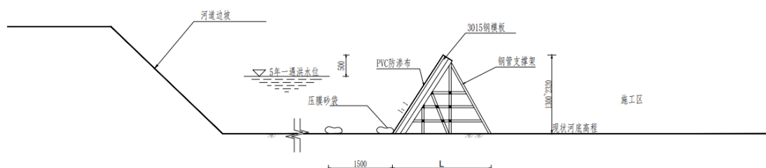
图 3-3 围堰断面示意图
