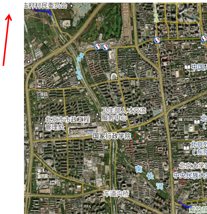
图 5 疏浚范围示意图
