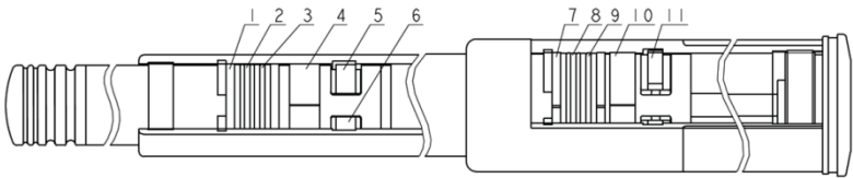
图2 内部主要零部件示意图
