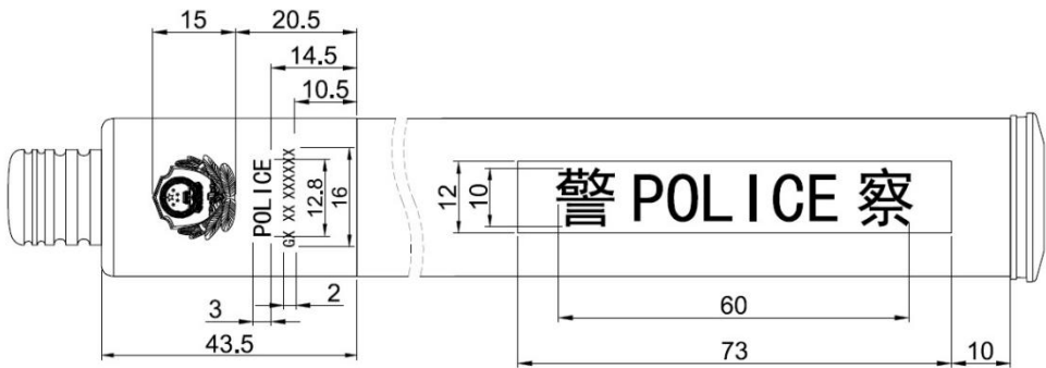
图4 伸缩警棍标识示意图
