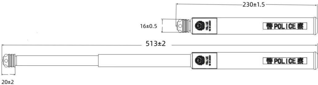
加强型尺寸
