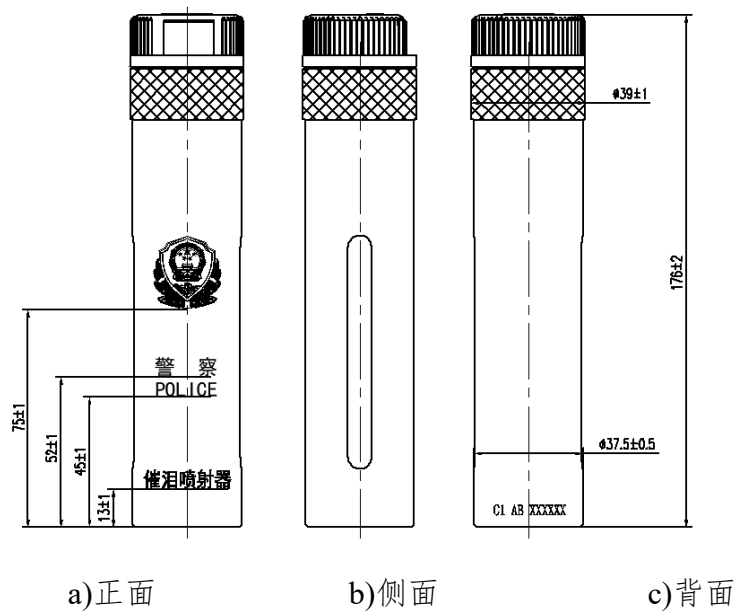
图 3 C1 催泪喷射器外形尺寸示意图 单位为毫米
