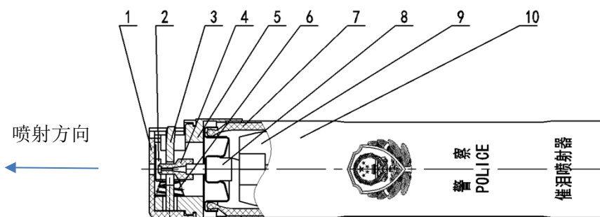
图1 横喷型催泪喷射器结构示意图
