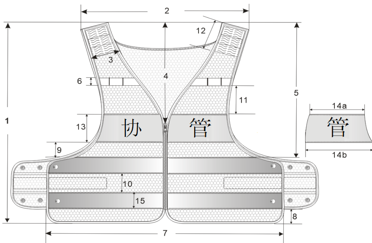
图 2a 反光背心成品尺寸测量方法
