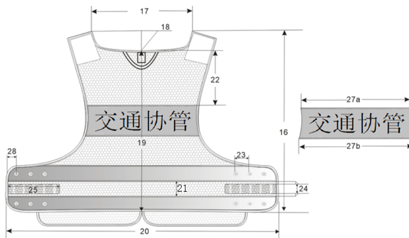
图 2b 反光背心成品尺寸测量方法
