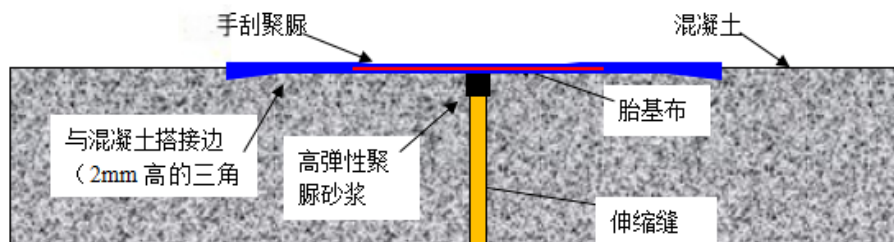
图 5.4.8-1 混凝土伸缩缝防渗处理示意图
