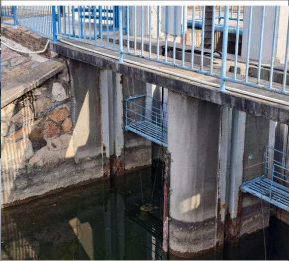
土城泄洪闸闸墩现状
