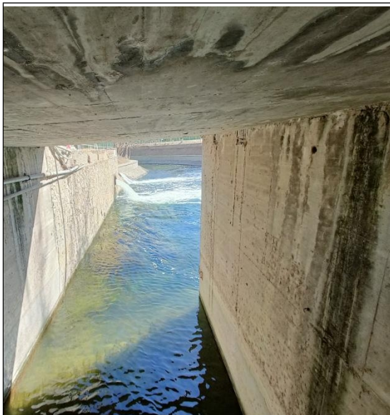
安河泄洪闸混凝土缺陷现状
