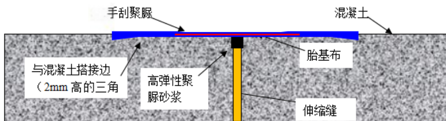
图 5.1.1 混凝土伸缩缝防渗处理示意图
