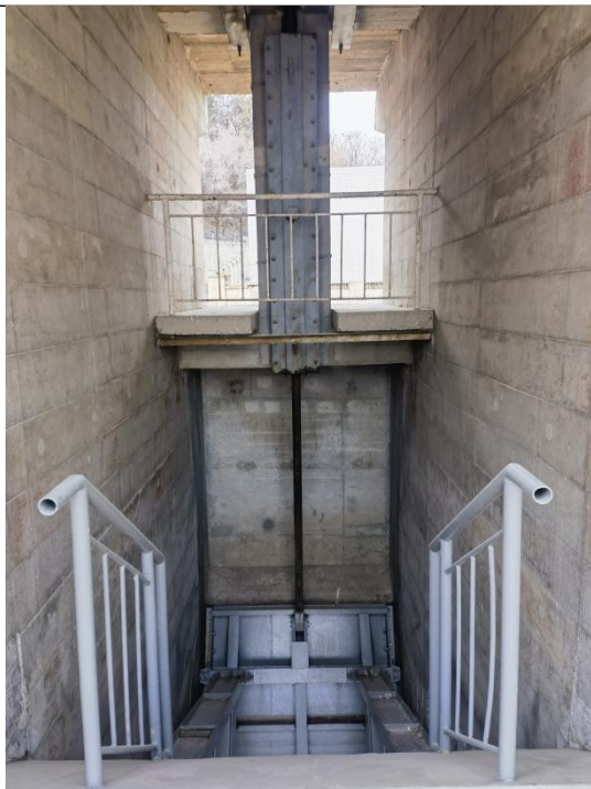
隧洞出口闸现状（三）
