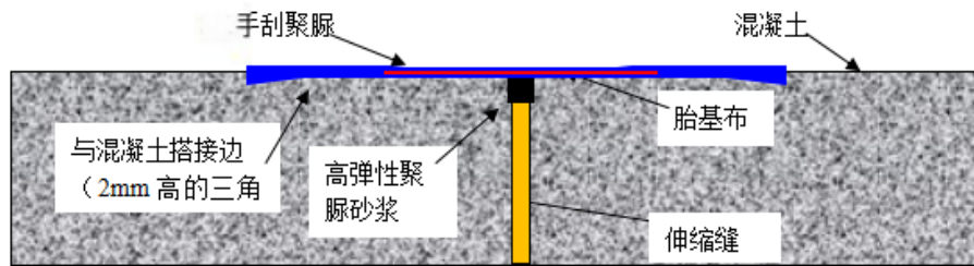
图 5.4.8-1 混凝土伸缩缝防渗处理示意图
