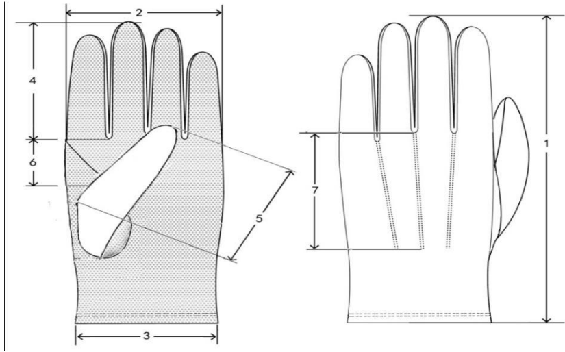
白针织手套（防滑胶粒）测量部位及编号示意图
