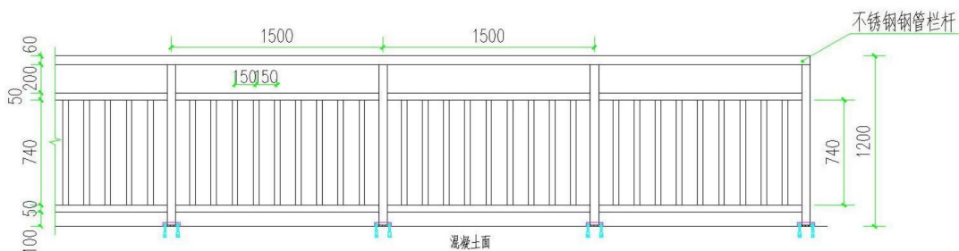
1.2m不锈钢栏杆立面图
