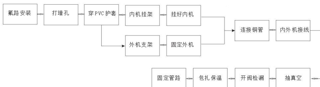
分体机氟路安装流程图
