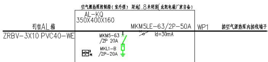
空气源热泵电气系统图
